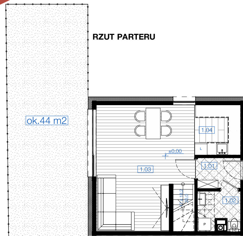
ZESTAWIENIE POWIERZCHNI - RZUT PARTERU
