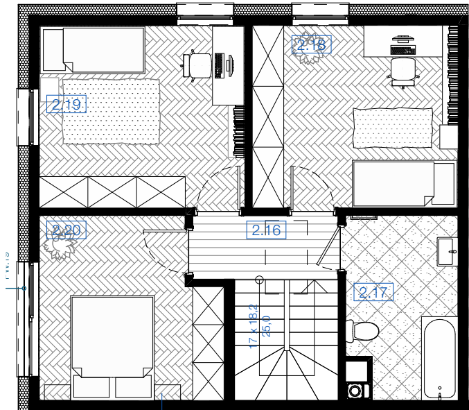
RZUT PIĘTRA
