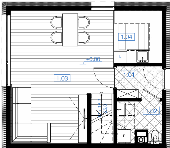
RZUT PARTERU
